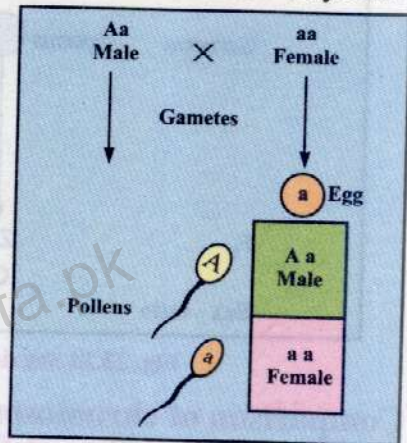
Fig. 22.24 Pollens determine Sex
