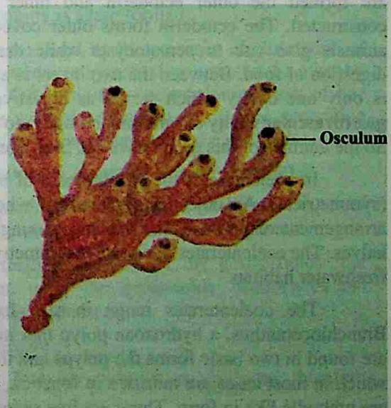
Fig. 10.4 Sycon
