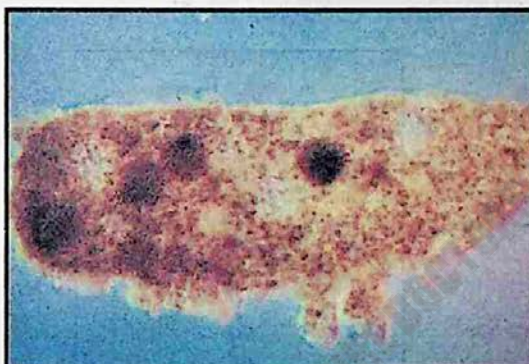
Pelomyxa palustris
