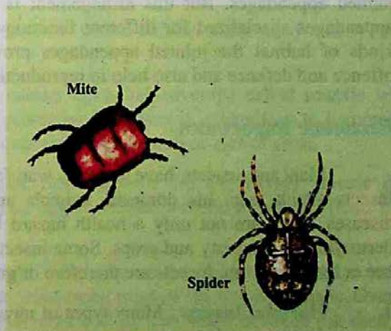
Fig. 10.10 Arachnids
