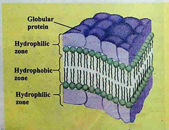
Fig. 4.4. Unit membrane
