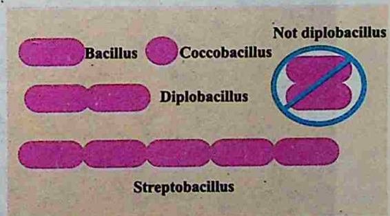
Fig. 6.3 Bacilli
